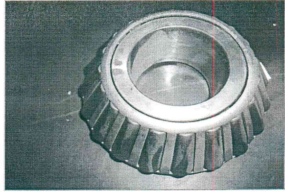
ROLAMENTO DO PINHÃO "B"
