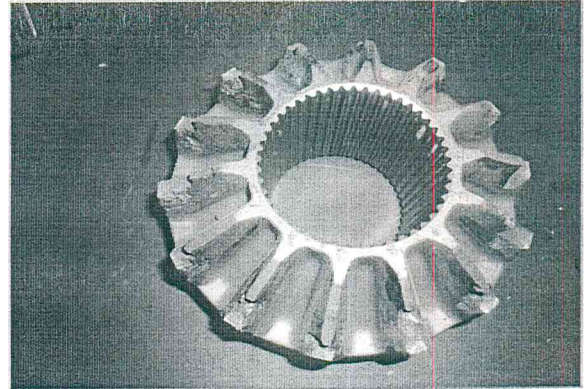
CAIXA SATÉLITE DESMONTADA - DETALHE DE COMPONENTE AVARIADO
