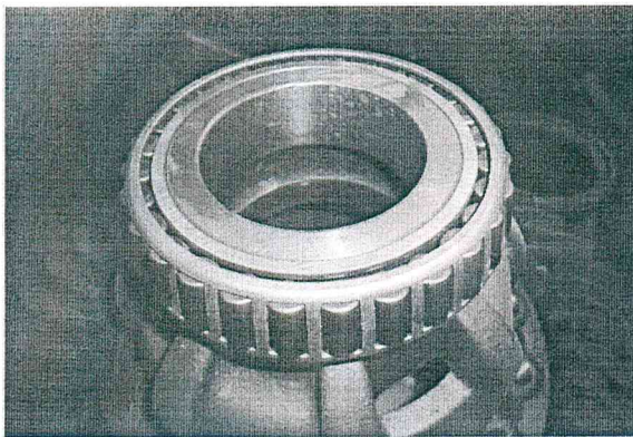
ROLAMENTO DA COROA "A"
