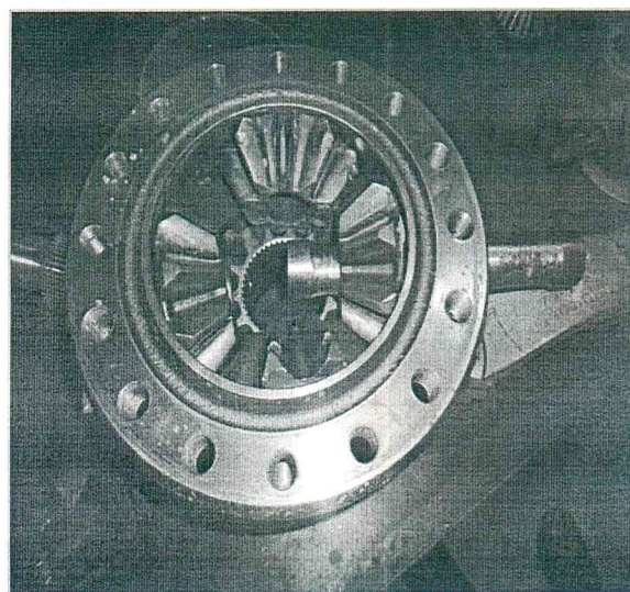
DETALHE DA CAIXA SATÉLITE MONTADA COMPLETA
