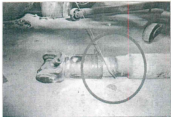
DETALHE DO EIXO CARDÃ, PARTE EM AZUL POSSIVELMENTE NÃO ESTAVA FAZENDO O MOVIMENTO CORRETO OCASIONANDO ASSIM ESFORÇO MAIS ELEVADO AO SISTEMA
