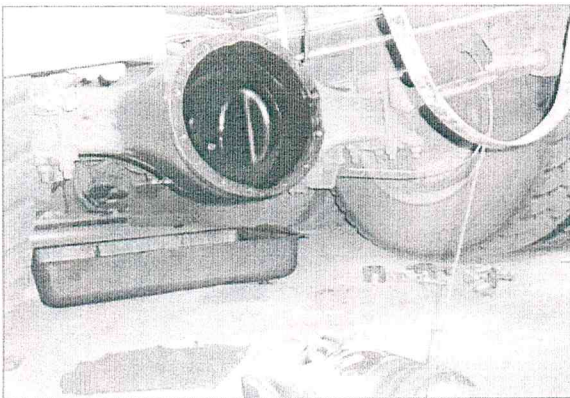
DETALHE DO CAMINHÃO BASCULANTE COM CONJUNTO DIFERENCIAL DESMONTADO
