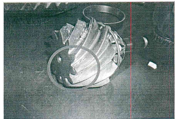
PINHÃO BEM AVARIADO (QUEBRADO E DESGASTADO)
