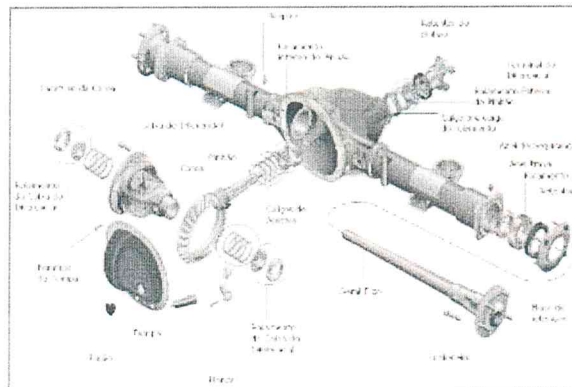
CONJUNTO DE DIFERENCIAL ILUSTRATIVO
