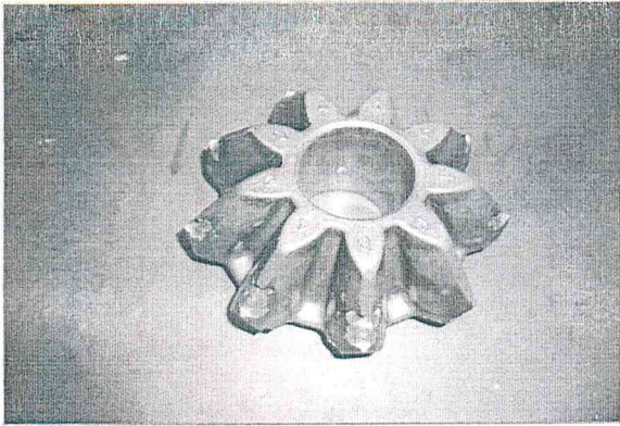
CAIXA SATÉLITE DESMONTADA - DETALHE DE COMPONENTE AVARIADO
